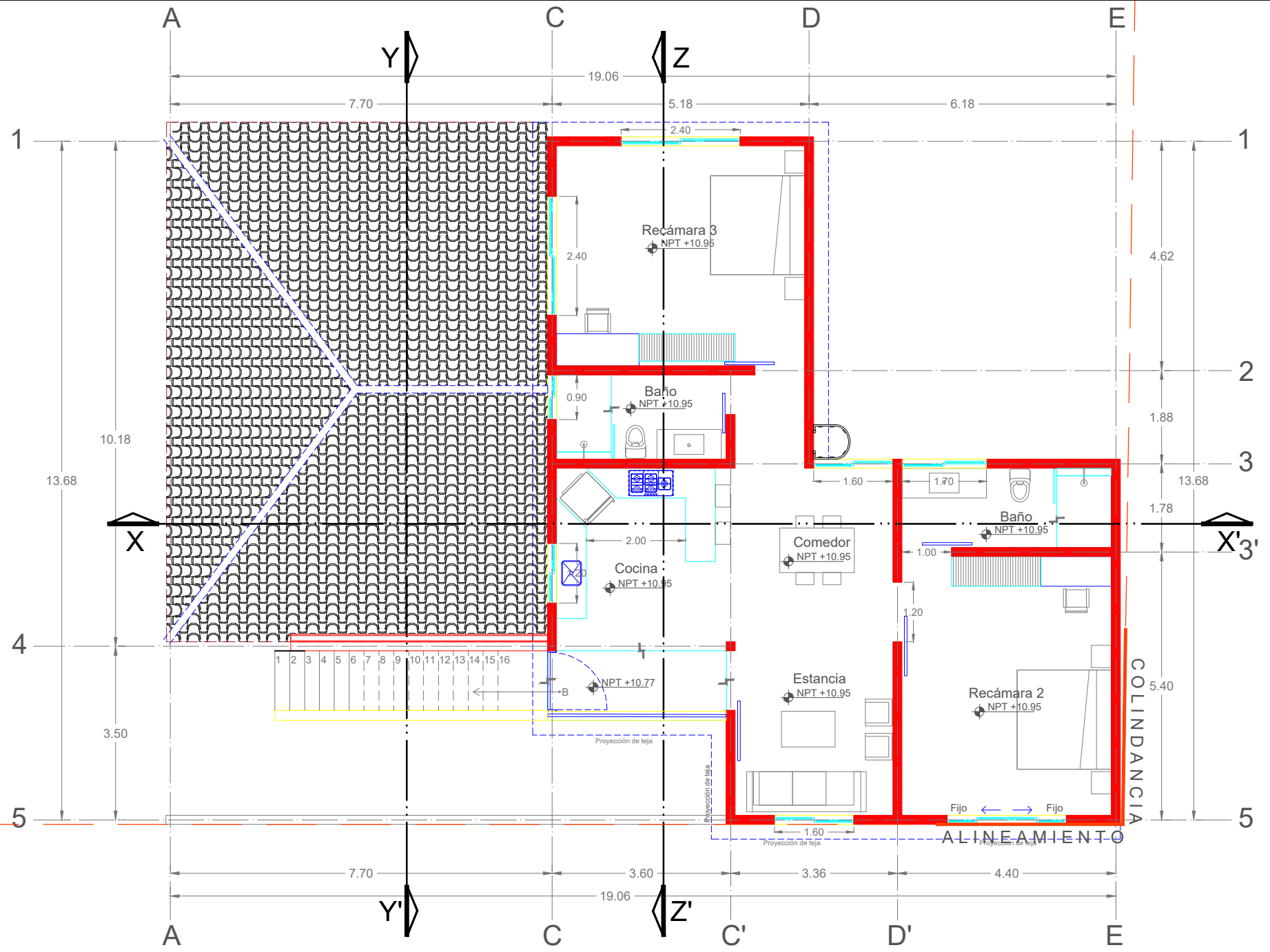
PLANTA ALTA
